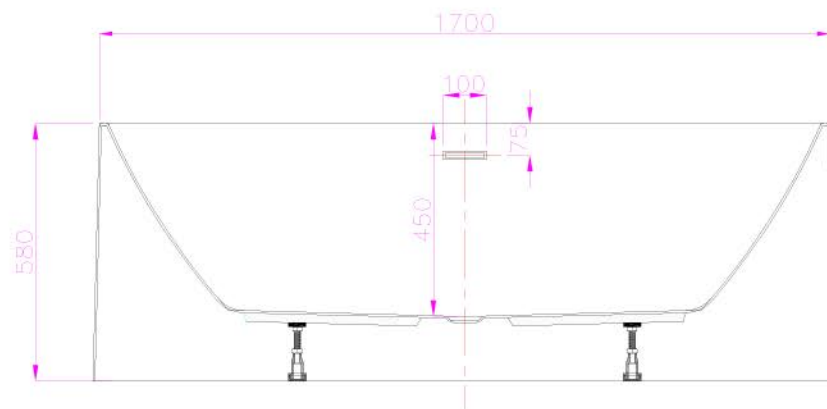
SEZIONE G-G
