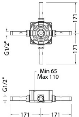
DISEGNO - DRAWING
